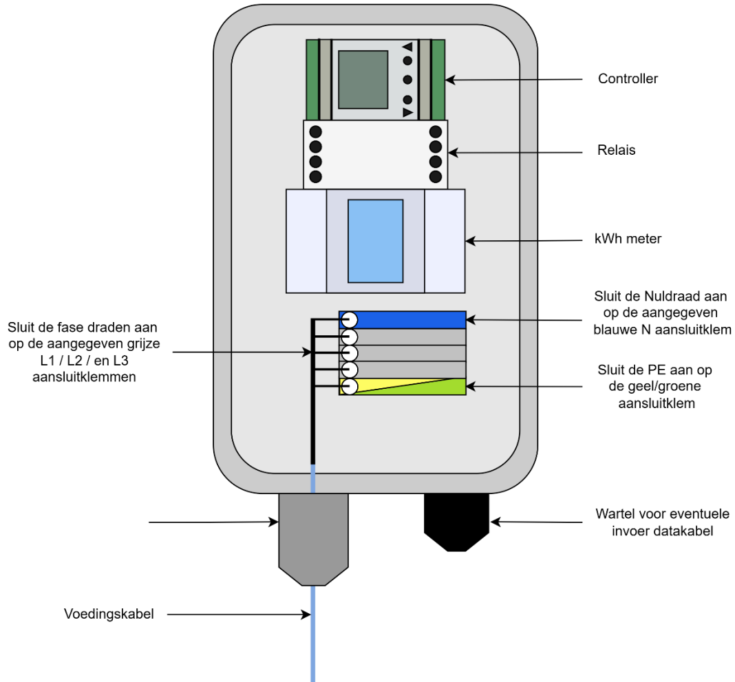
Figuur 3 aansluiting voedingskabel enkelvoudige laadpaal
