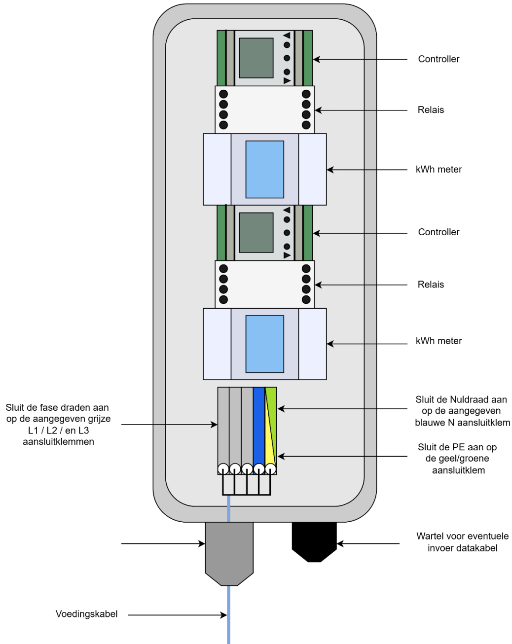
Figuur 4 aansluiting voedingskabel dubbele laadpaal
