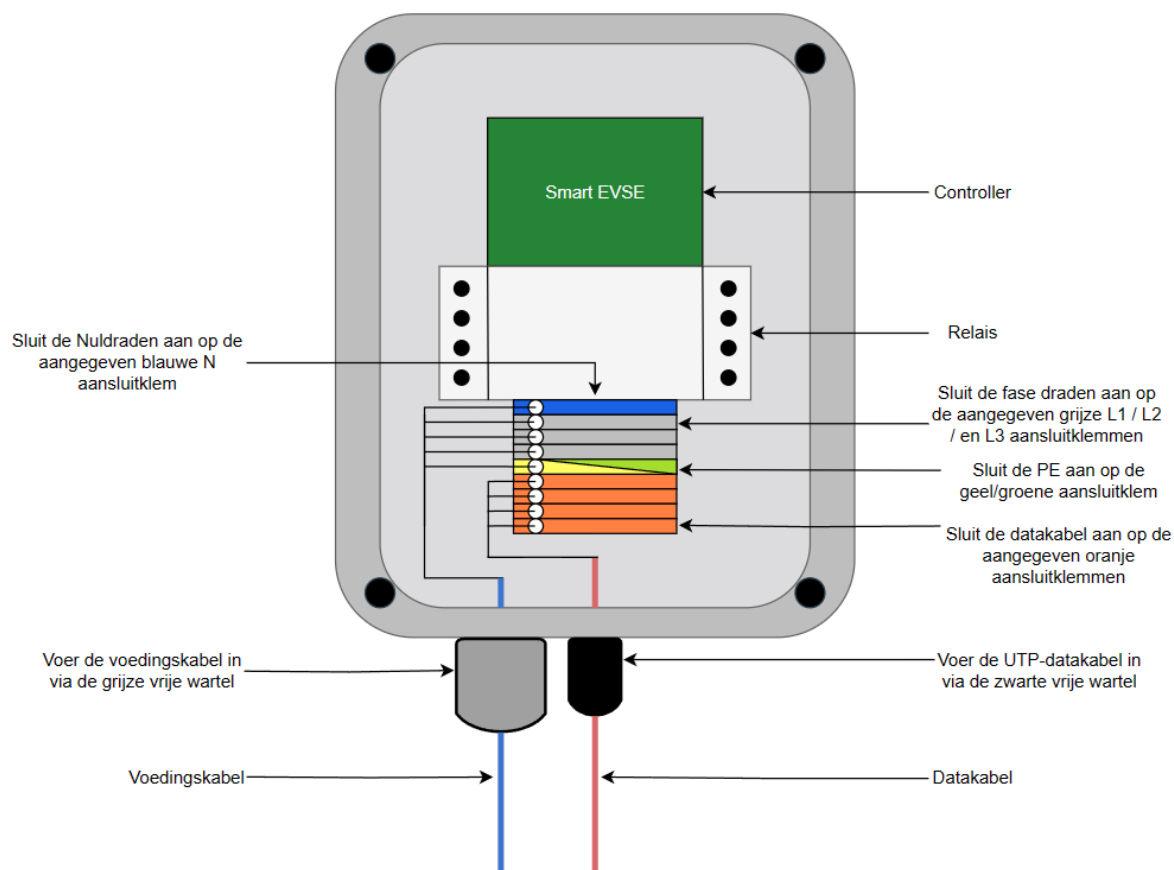
Figuur 3 aansluiting voedingskabel laadpaal
